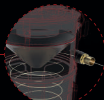
Boca tangencial con ciclón
