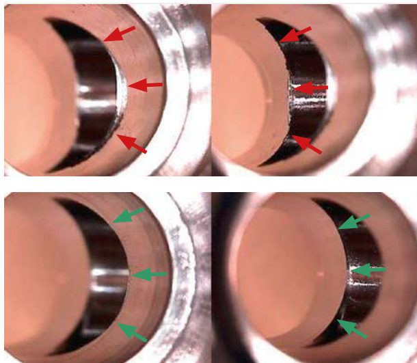
Imagen 1: El canto del agujero está limpio y libre de rebaba. Parte superior: Antes de rebado. Parte inferior: Después de rebado.
