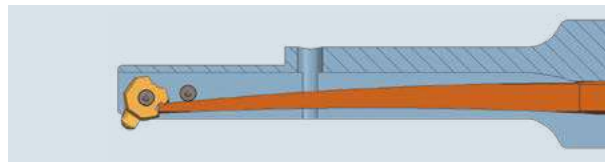
Imagen 3: El fleje precargado y el mango rebado permite el rebado de agujeros con alto grado de irregularidad.
