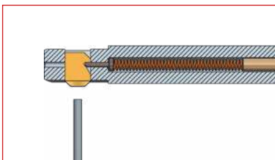
SNAP- Herramienta con la cuchilla montada
