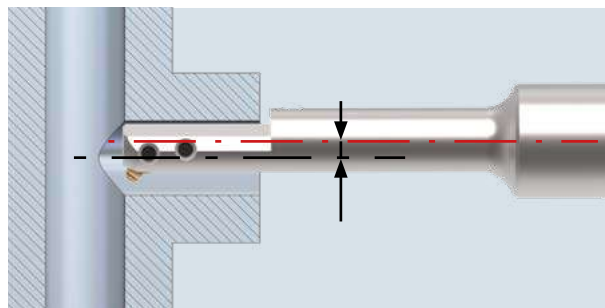
Imagen 2: El acceso de herramienta a la zona de rebado se hace a través del agujero transversal.
