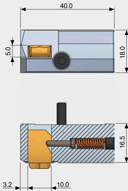
Cartucho SNAP20 > Ø35.0 mm
