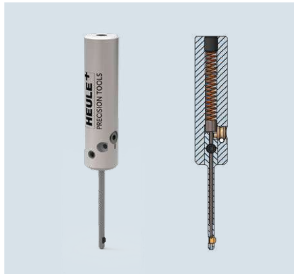
Imagen: SNAP2- El diseño de la herramienta se compone de dos partes, por razones de tamaño: el cuerpo de la herramienta y la carcasa de la cuchilla.
