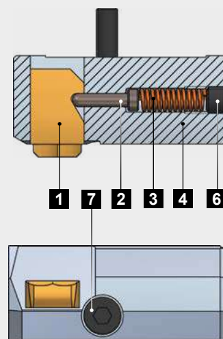
Cartucho SNAP20 > Ø35.0 mm
